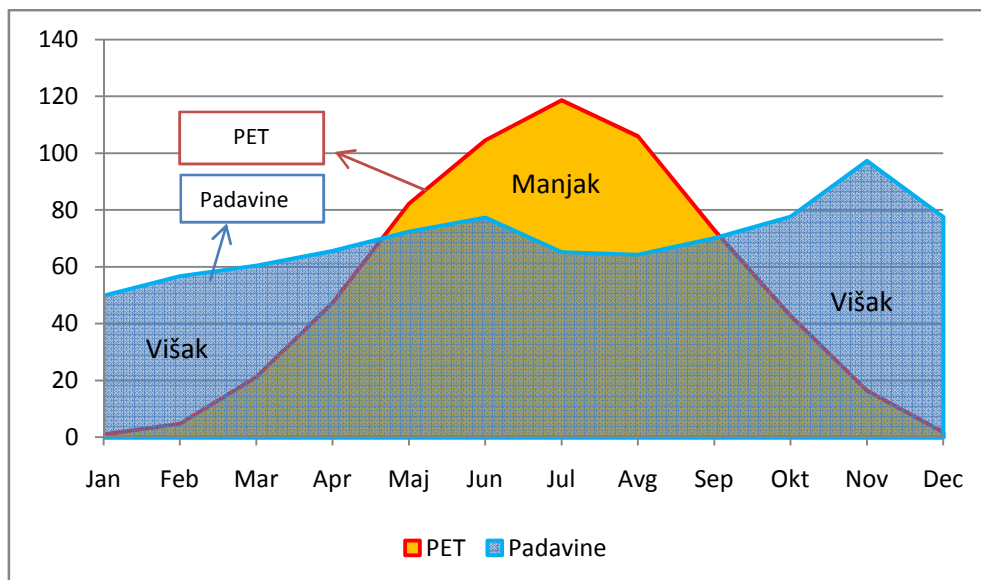
Grafikon 3. Srednji vodni bilans za područje Travnika – Pri RLPV 100 mm
