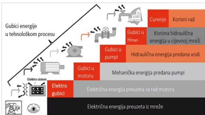
Sveobuhvatno sagledavanje gubitaka energije u tehnološkom procesu
